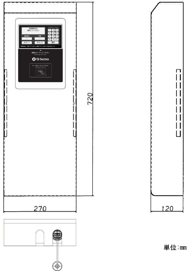
図 2-1 外観図
