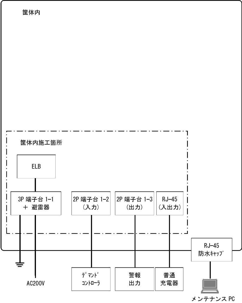
図 5-1 インターフェース接続図
