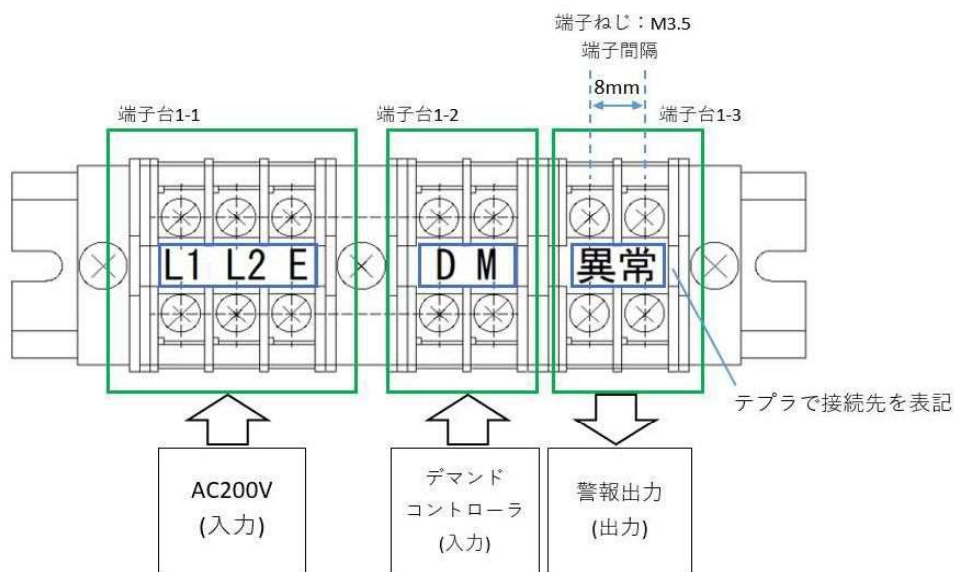
図 5-2 端子台
