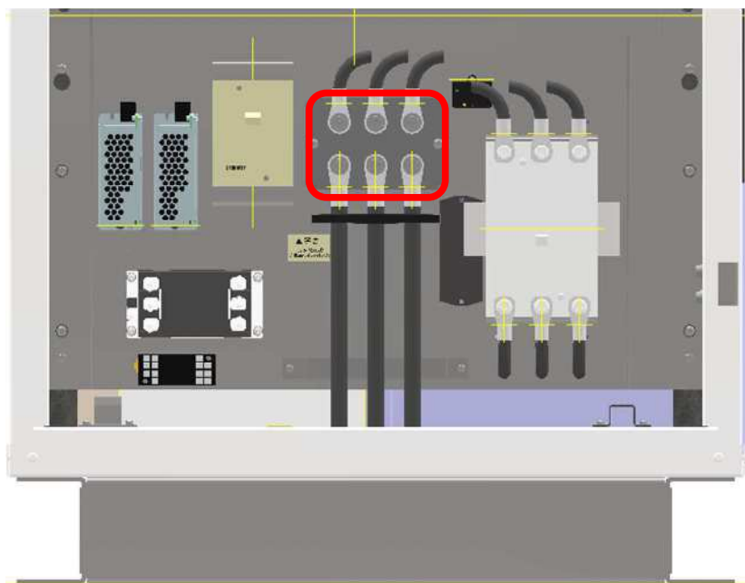
図 8. 端子台の保護カバー
