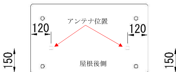
図 11. 屋根へのアンテナ取付け位置寸法
