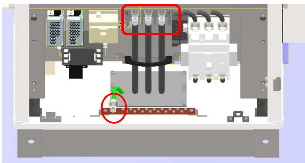
図 9. ケーブル接続用端子
