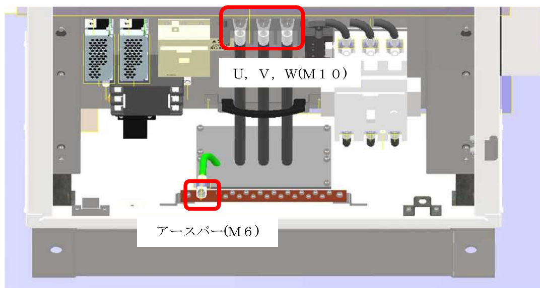
図 10. ケーブル接続箇所
