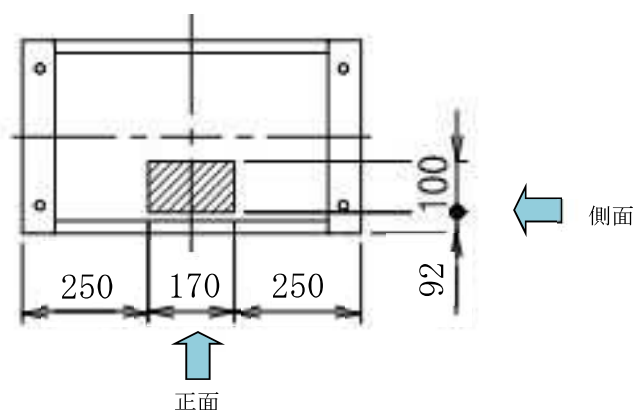
図4. ケーブル入線口の位置
