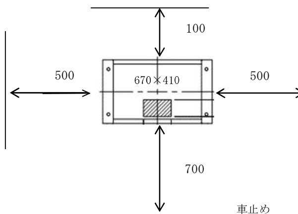
図5. 保守スペース
