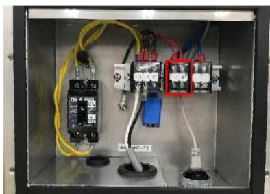
デマンドコントローラーからの信号線
