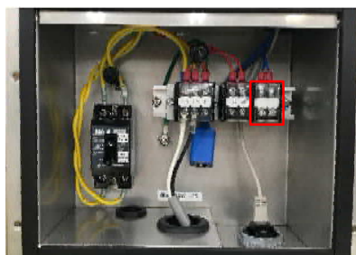
この端子はモデルに応じて使い方が異なります 違いは左図を参照下さい
